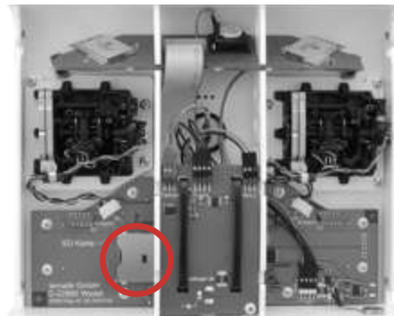
SD-Kartenslot im Sender
