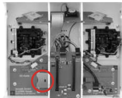
SD-Kartenslot im Sender
